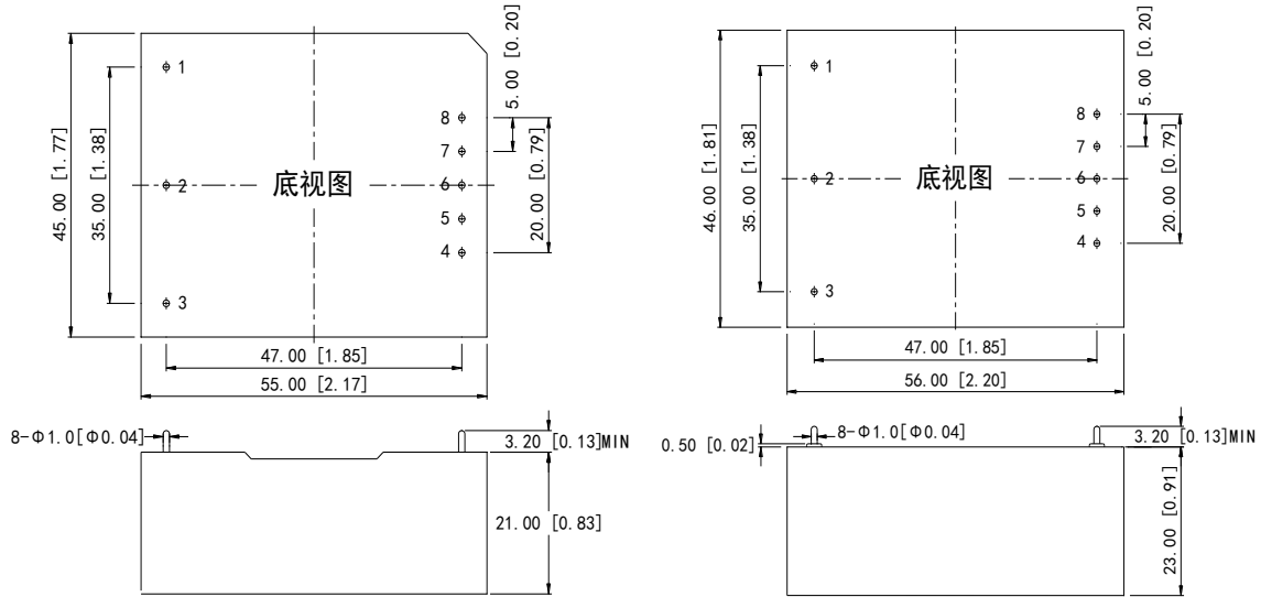
塑料壳尺寸
